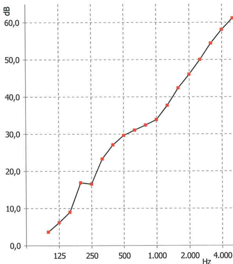
Reducción del nivel de presión acústica de ruido de impactos, \Delta L
